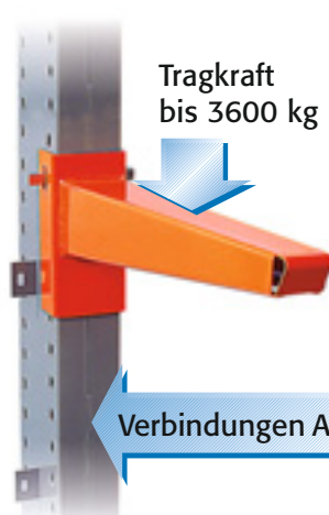
Abmessungen und Belastungsübersicht der ELVEDI-Schwerlast-Freitrageregale
