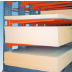
Grosse Fachhöhe für bequeme Ein- und Auslagerung.
