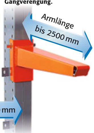
Abmessungen und Belastungsübersicht der ELVEDI-Schwerlast-Freitrageregale
