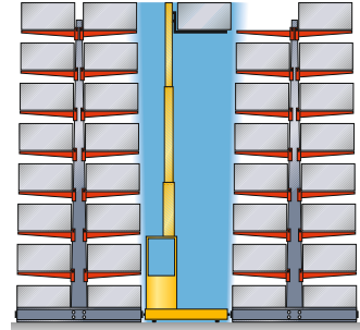
Konisch zulaufende Ständer für bessere Höhensicht und bestmögliche Arbeitssicherheit – ohne Gangverengung.
